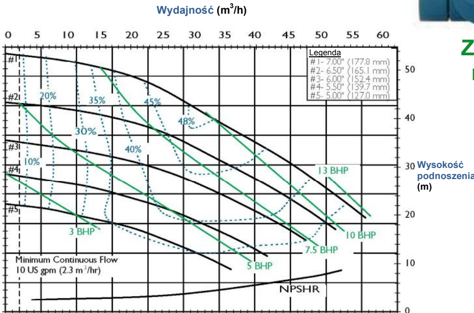
SP22 WYDAJNOŚĆ przy wolnym napływie 3450 RPM
